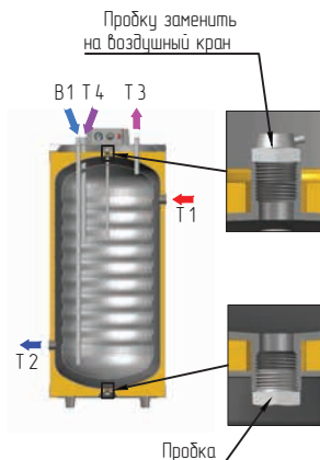
Рис. 5 Напольный монтаж
